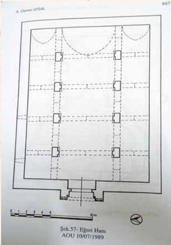
Eğret Hanı Planı (A.O. Uysal'dan)
