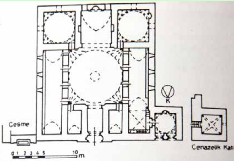
Çizim 2 : Ebû'l-Mücahid Yusuf Medresesi, rölöve planı.
