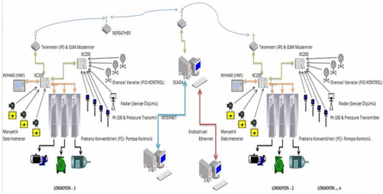
Afjet otomasyon sistem mimarisi
